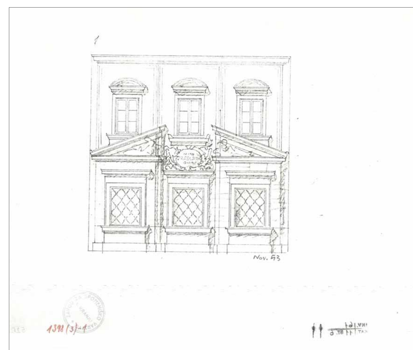
Načrt arhitekta Jožeta Plečnika za prenovu Prešernove hiše iz leta 1953 (Arhiv ZVKDS OE Kranj)
