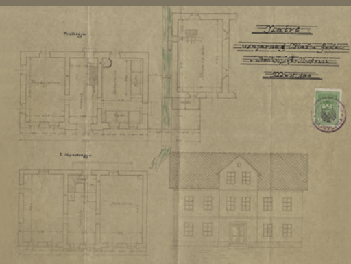
Načrt Godčeve usnjarne iz leta 1927
