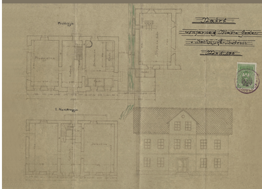
Načrt Godčeve usnjarne iz leta 1927
